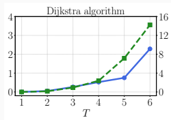
(b) Dijkstra
